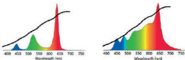
RGB (W) vs. 6カラーの比較:アンバー、シアン、ライムを加えることで、RGB (W) システムで見られる波長のギャップを補完し、より完璧なカラー再生を実現します。
